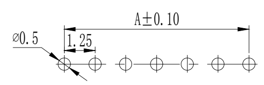
P.C.B LAYOUT
